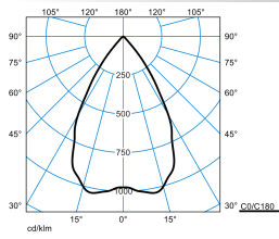
InperiaLP C05 HR19 1000-830 ET 03
