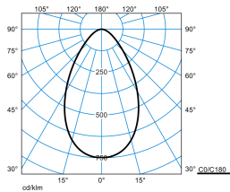
InperiaLP C05 HR19 1000-830 03 + DA-M 01
