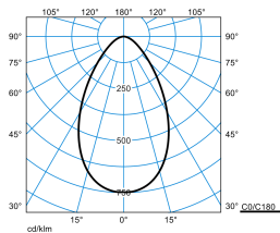
InperiaLP C05 HR19 1000-830 03 + DA-M 03
