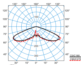
Publisca P1-RB6L-LR/2000-740 3G1S ET (CLO end value)
