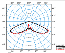
Publisca P1-RB6L-LR/2000-740 3G1S TX047629 DIN 5040: A20 UTE: 1,00 J DLOR: 100 % ULOR: 0 % CEN Flux Code: 20 57 98 100 100
