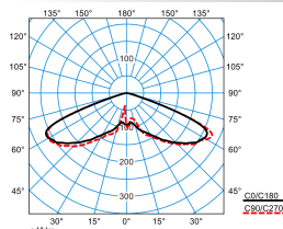
Publisca P1-RB6L-LR/2000-740 3G1S ET (CLO initial value)
