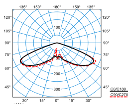
Publisca P1-RB6L-LR/2000-740 3G1S ET (CLO end value) TX301026 DIN 5040: A20 UTE: 1,00 J DLOR: 100 % ULOR: 0 % CEN Flux Code: 20 57 98 100 100
