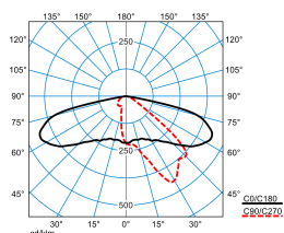
Cuvia40-AB2L4S3-21-7TW-ET-CAB-26 (DSU-CLO initial value)
