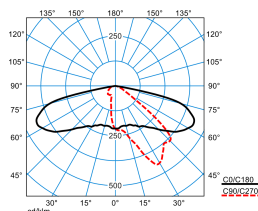
Cuvia40-AB2L4S3-21-7TW-ET-CAB-26 (DCW-CLO end value)
