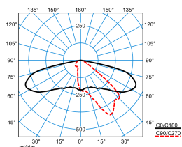
Cuvia40-AB2L4S3-21-7TW-ET-CAB-26 (DSU-CLO end value)
