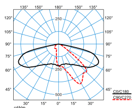
Cuvia40-AB2L4S3-21-7TW-ET-CAB-26 (DWW-CLO end value)
