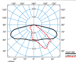
LIQ 50-AB2L/5600-740 6G1S ET TX776317 DIN 5040: A30 UTE: 1,00 G DLOR: 100 % ULOR: 0 % CEN Flux Code: 36 71 96 100 100
