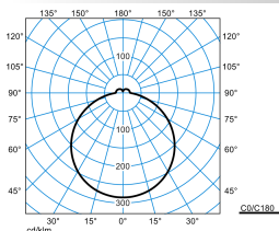
Olisq RWD2 DW 40-8TW ETDD8 IP54 (DWW)
