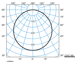
Olisq RWD2 DW 40-8TW ETDD8 IP54 + RWD2 ZDR 1/1 05 (DWW)
