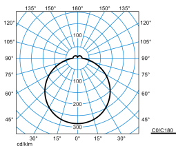
Olisq RWD2 DW 40-8TW ETDD8 IP54 (DSU)
