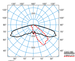
Publisca P1W-AB2L-LRA/3200-740 4G1S ET (CLO end value)
