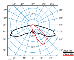
Publisca P1W-AB2L-LRA/3200-740 4G1S ET (CLO initial value)
