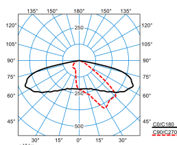
LIQ 50N-AB2L-LR/2200-740 4G1 ET (CLO end value)
