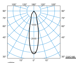
E-Line PRO 78 BV G2 RF-MF 20-835 M34 ET 01 Blank
