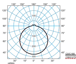
Olisq QWD2 DW 35-8TW ETBLE +CAS IP54 (DSU)
