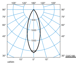
Amatris QC1 SRRFL 4-9MC ET 05 2KIT + HC-19 05 (stage 2)
