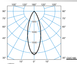
Amatris QC1 SRRFL 4-9MC ET 05 2KIT + HC-19 05 (stage 1)
