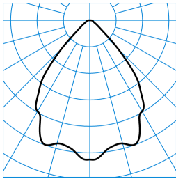
InperiaLP C05 HR22 1000-840 01 + ZN-PC TX041688 ■ C0 - C180
