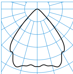
InperiaLP C05 HR22 1000-840 01 + DA 01 TX041682 ■ C0 - C180
