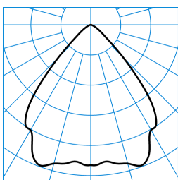
InperiaLP C05 HR22 1000-840 01 + RD-PC TX041686 ■ C0 - C180
