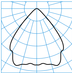
InperiaLP C05 HR22 1000-840 01 + RG-PC TX041687 ■ C0 - C180
