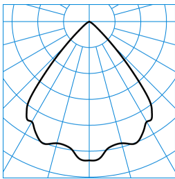
InperiaLP C05 HR22 1000-840 ETDD 01 TX768308 ■ C0 - C180 ■ C90 - C270
