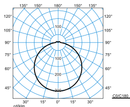
Olisq RWD2 DW 40-830 ET EB3 + Olisq RWD2 ZDR 1/2 03 TX427778
