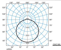
Olisq RWD2 DW 40-830 ET EB3
