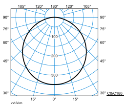
Olisq RWD2 DW 40-830 ET EB3 + Olisq RWD2 ZDR 1/1 01 TX425940
