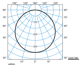
Olisq RWD2 DW 40-830 ET EB3 + Olisq RWD2 ZDR 1/1 01
