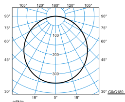
Olisq RWD2 DW 40-830 ET EB3 + Olisq RWD2 ZDR 1/1 03
