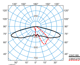
Publisca P1W-AB2L-LRA/2600-730 3G1S ET (CLO end value)
