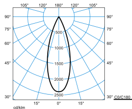
7651 Lentyp L-FL 40-827 M32 ET 05 (150)
