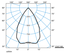
InperiaLP C05 HR19 1800-840 ET 03 TX768161
