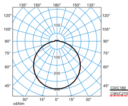
Olisq QWD3 DW 30-840 ETBLE +DMM IK + Olisq QWD3 ZDR 1/2 01
