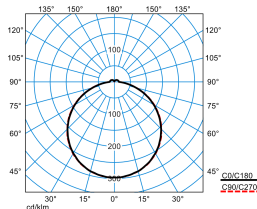
Olisq QWD3 DW 30-840 ETBLE +DMM IK + Olisq QWD3 ZDR 1/2 03
