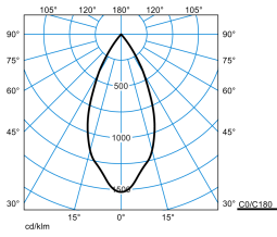
E-Line PRO 78 BV G2 RF-WFL 30-BC M49 ETDD 01 TX717321
