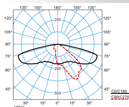
9301K AB2L-LR-SLR1/4600-730 8G3 ET (CLO initial value)
