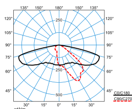
9301K AB2L-LR-SLR1/4600-730 8G3 ET (CLO end value)
