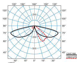
LTX P-AB2L-LRA/15/18/26-740 4G1 (2600 lm)
