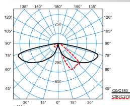
LTX P-AB2L-LRA/15/18/26-740 4G1 (1500 lm)
