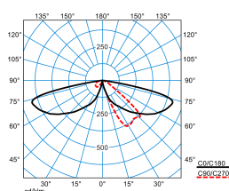
LTX P-AB2L-LRA/15/18/26-740 4G1 (1800 lm)
