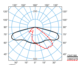
LnPlus 60-AB7L/26000-740 24G1 ETDD (CLO end value)
