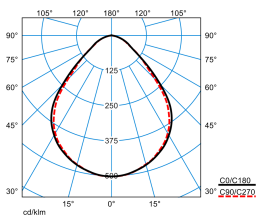
Opendo D1-L PW19 20-36/4/ML-840 ET 03 (2800lm) TX376523
