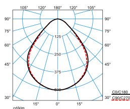
Opendo D1-L PW19 20-36/4/ML-840 ET 03 (2800lm)
