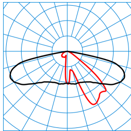
Publisca P2-AB2L/1100-730 2G1S TX047696 ■ C0 - C180 ■ C90 - C270 DIN 5040: A30 UTE: 1,00 G DLOR: 100 % ULOR: 0 % CEN Flux Code: 34 70 96 100 100
