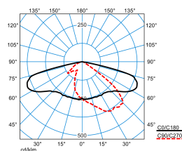
LIQ 70N-AB7L-LRA/6800-740 8G1 ETDD(CLO end value)
