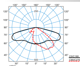
LIQ 70N-AB7L-LRA/6800-740 8G1 ETDD(CLO initial value)
