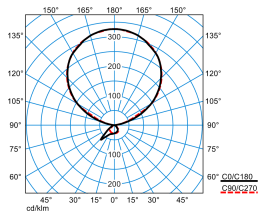
Luceos S-U PAW-IL 300-840 ETDD 01 (LEO2) TX877124
