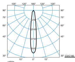
E-Line PRO 78 BV G2 RF-SP 30-840 M35 ET 05 Blank
