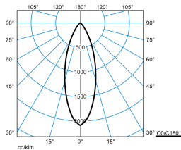
Amatris RC2 SRRFL 8-9MC ET 05 2KIT + HC-19 05 (stage 2)
