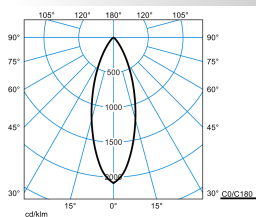
Amatris RC2 SRRFL 8-9MC ET 05 2KIT + HC-19 05 (stage 1)
