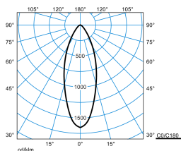
Amatris RC2 SRRFL 8-9MC ET 05 2KIT + PC IP54 (stage 2)
