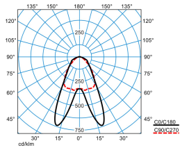
ELINE LDAN100 830 L150 1 20
