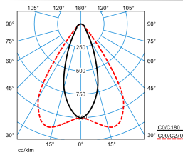
7651IP MironaF HR 270-840ETDD L225 01ESG (LEO3)
