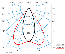
7651IP MironaF HR 270-840ETDD L225 01ESG (LEO1)
