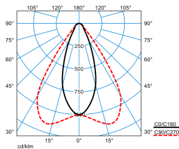
7651IP MironaF HR 270-840ETDD L225 01ESG (LEO2)
