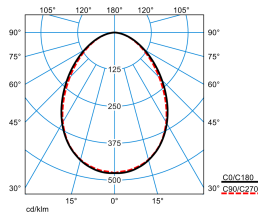
SFlow C1-L MRWD LED3200-840 ET 01 TX771461
