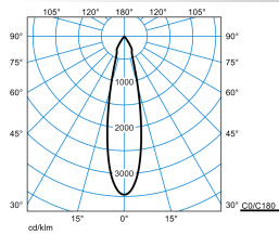
KaloP 3P RF-MF 50-830 M41 ETDD 05
