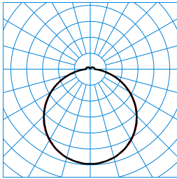
Olisq QWD3 DW 45-840 ETDD IP54 + Olisq QWD3 ZDR 1/2 01 TX461681
