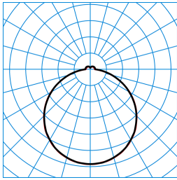
Olisq QWD3 DW 45-840 ETDD IP54 TX375745
