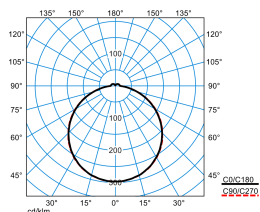
Olisq QWD3 DW 45-840 ETDD IP54 + Olisq QWD3 ZDR 1/2 05 TX461953
