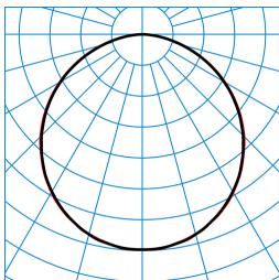
Olisq QWD3 DW 45-840 ETDD IP54 + Olisq QWD3 ZDR 1/1 01 TX460811
