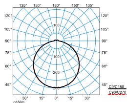
Olisq QWD3 DW 45-840 ETDD IP54 + Olisq QWD3 ZDR 1/2 03 TX461300
