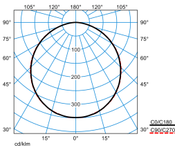
Olisq QWD3 DW 45-840 ETDD IP54 + Olisq QWD3 ZDR 1/1 03 TX460923
