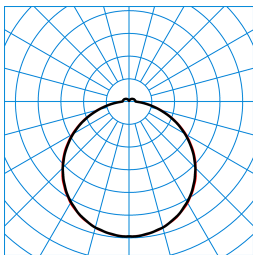
Olisq QWD3 DW 45-840 ETDD IP54 + Olisq QWD3 ZDR 1/2 05 TX461953
