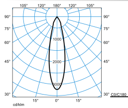
CaniloP 3P RF-MF 60-EW M50 ETDD 01
