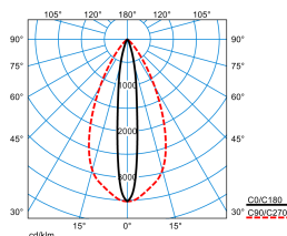
Altigo G2 C 60 SE6L/800-830 1G1P + G2 VE IP66 24V DC 30W
