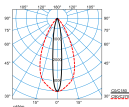
Altigo G2 C 60 SE6L/800-830 1G1P + G2 VE IP66 24V DC 80W
