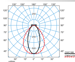
TugraHE 18 PN 64-840 ET IP69K 23
