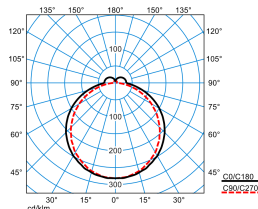
Olisq LWD1 DW 20-8TW ETDD8 IP54 IK (DCW)
