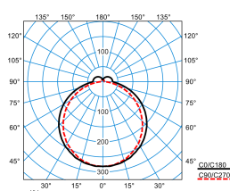
Olisq LWD1 DW 20-8TW ETDD8 IP54 IK (DSU)
