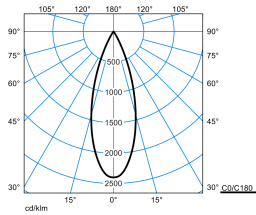
7651 Lentyp L-FL 40-827 M32 ET 01 (150)
