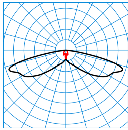
Publisca P2-SB3L/1000-730 2G1S TX047916 ■ C0 - C180 ■ C90 - C270 DIN 5040: A30 UTE: 1,00 l DLOR: 100 % ULOR: 0 % CEN Flux Code: 31 65 93 100 100
