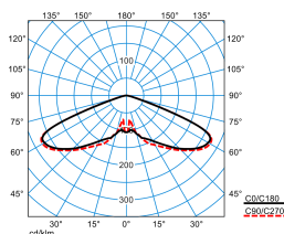
Publisca P1-RB6L-LR/4200-730 6G1S
