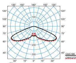
Publisca P1-RB6L-LR/4200-730 6G1S ET (CLO end value)
