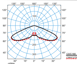
Publisca P1-RB6L-LR/4200-730 6G1S ET (CLO initial value)
