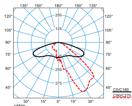
Publisca P1-AB2L-LR/3500-730 4G1S ET (CLO initial value)
