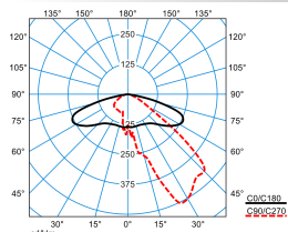
Publisca P1-AB2L-LR/3500-730 4G1S
