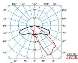
Publisca P1-AB2L-LR/3500-730 4G1S ET (CLO end value)
