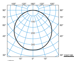
Olisq RWD1 DW 20-840 ET IP54 PC + Olisq RWD1 ZDR 1/1 01
