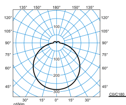
Olisq RWD1 DW 20-840 ET IP54 PC + Olisq RWD1 ZDR 1/2 03
