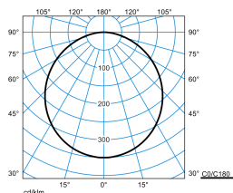
Olisq RWD1 DW 20-840 ET IP54 PC + Olisq RWD1 ZVF 05
