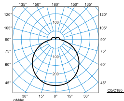
Olisq RWD1 DW 20-840 ET IP54 PC
