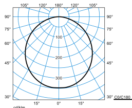
Olisq RWD1 DW 20-840 ET IP54 PC + Olisq RWD1 ZDR 1/1 05
