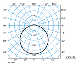
Olisq RWD1 DW 20-840 ET IP54 PC + Olisq RWD1 ZDR 1/2 01
