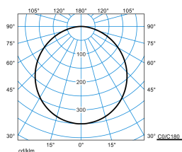
Olisq RWD1 DW 20-840 ET IP54 PC + Olisq RWD1 ZVF 01
