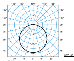
Olisq RWD1 DW 20-840 ET IP54 PC + Olisq RWD1 C 01
