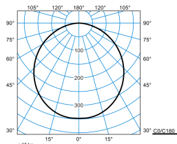
Olisq RWD1 DW 20-840 ET IP54 PC + Olisq RWD1 ZDR 1/1 03
