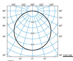
Olisq RWD2 DW 14-40/4/ML-840 ET PC + Olisq RWD2 ZVF 05 (stage 3)
