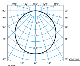
Olisq RWD2 DW 14-40/4/ML-840 ET PC + Olisq RWD2 ZDR 1/1 01 (stage 1)
