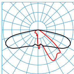
Publisca P2-AB2L/2000-730 3G1S ETDD (CLO initial value) TX300500 ■ C0 - C180 ■ C90 - C270 DIN 5040: A30 UTE: 1,00 l DLOR: 100 % ULOR: 0 % CEN Flux Code: 34 71 96 100 100
