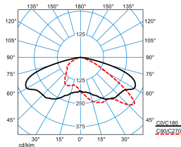
LnPlus 40-AB7L-LR/3200-722 4G1 ET (CLO end value)
