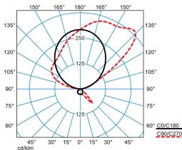
Luceos S G3 PAW-IA 170-9TW ETDS FU 05 (DCW)
