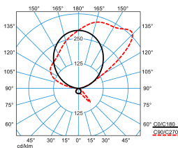
Luceos S G3 PAW-IA 170-9TW ETDS FU 05 (DSU)
