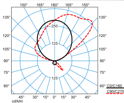
Luceos S G3 PAW-IA 170-9TW ETDS FU 05 (DWW)
