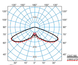
Publisca P1-RB6L-LRA/3500-730 4G1S ET (CLO end value)
