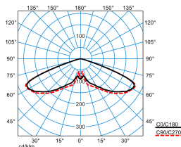
Publisca P1-RB6L-LRA/3500-730 4G1S
