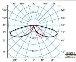
LTX KT-AB2L-LRA/1200-730 2G1 ETDD
