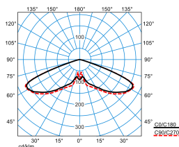
Publisca P2-RB6L-LR/3500-740 4G1S ET (CLO end value)
