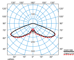
Publisca P2-RB6L-LR/3500-740 4G1S ET (CLO initial value)
