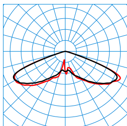
Publisca P1-RB6L-LRA/2600-740 3G1S ET (CLO end value) TX300806 ■ C0 - C180 ■ C90 - C270 DIN 5040: A20 UTE: 1,00 J DLOR: 100 % ULOR: 0 % CEN Flux Code: 20 57 98 100 100
