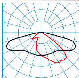
LnPlus 60-AB7L-SLR1/35000-740 24G1 ET (CLO end value) TX390200
