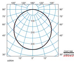
Olisq QWD3 DW 30-830 ETBLE +DMM IP54 IK + Olisq QWD3 ZDR 1/1 03
