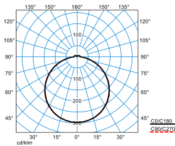
Olisq QWD3 DW 30-830 ETBLE +DMM IP54 IK + Olisq QWD3 ZDR 1/2 03
